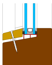
Systeem 3 A
